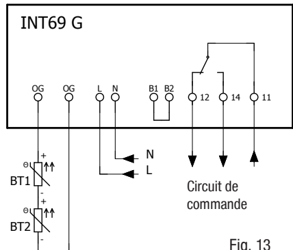
Fig. 13 Boîte à bornes
