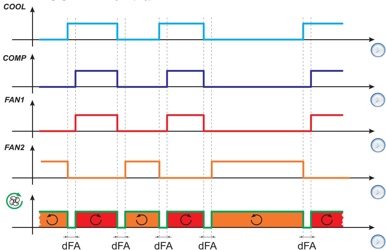
Schéma de réglage en modalité nuit (Night)
