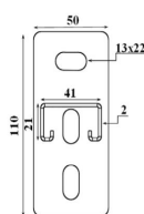
Console 41 x 21 - schéma technique
