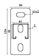
Console 41 x 41 - schéma technique
