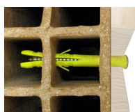
Cheville CQLV - vue en coupe dans la brique
